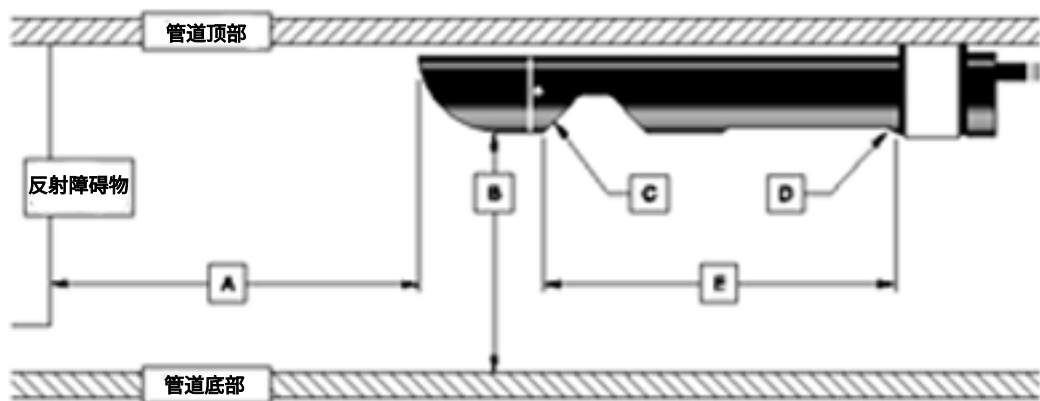
图 38 管道侧视图
